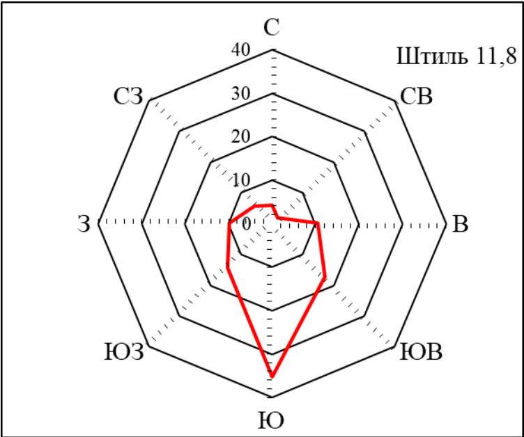
Рисунок 4.2 – Повторяемость направления ветра за январь, МС Салым
