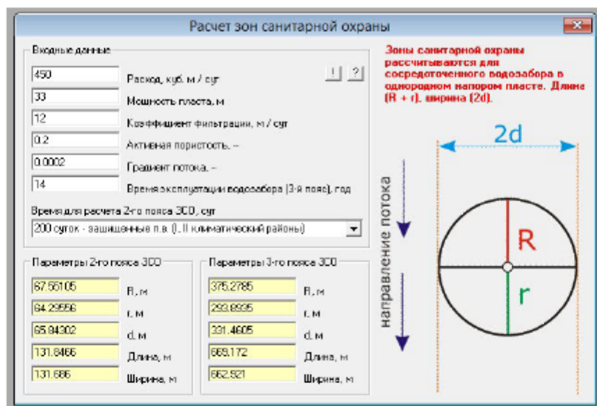
Рис. 7.1 – Расчет зон санитарной охраны водозабора подземных вод для атылского горизонта
