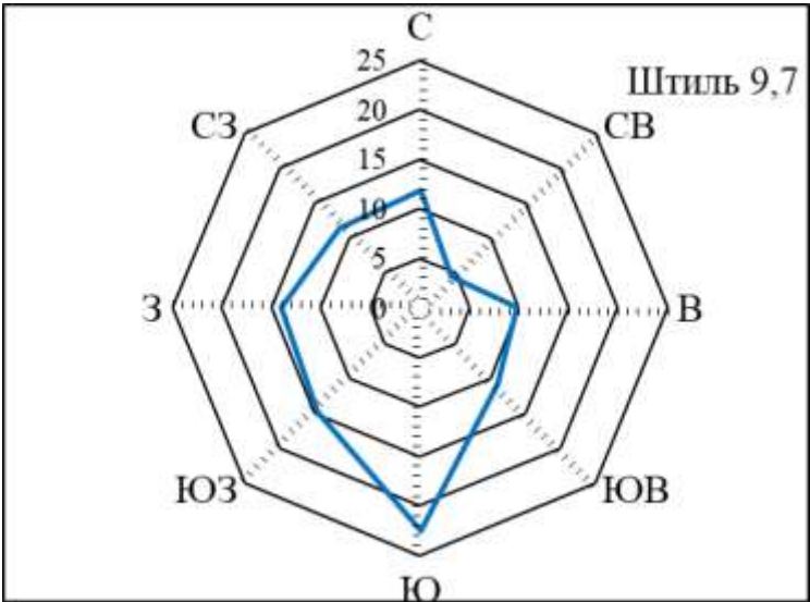
Рисунок 4.1 – Повторяемость направления ветра за год, МС Салым
